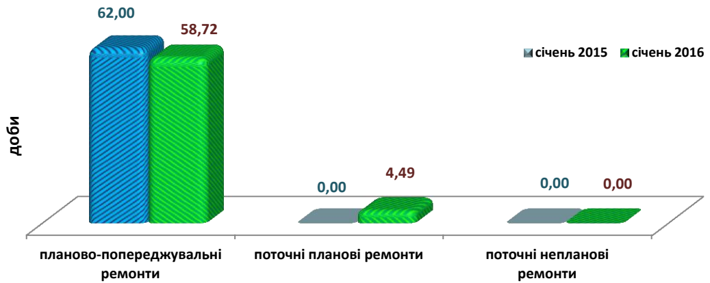
Рис. 5. Тривалість перебування енергоблоків АЕС у ремонтах
